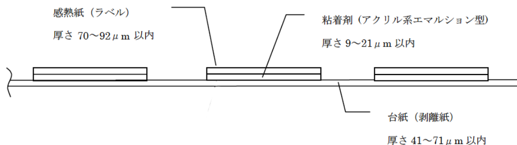
ダイカットラベル紙 厚さ条件図
