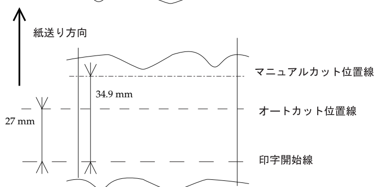
TM-U220 (A、B タイプ) (76mm ロール紙使用時)
