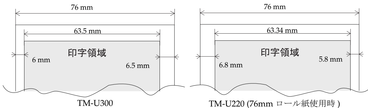
印字領域とマージン
