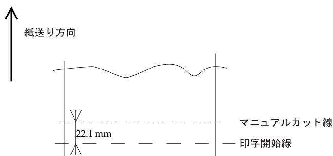
TM-U220 (Type D) (76mm ロール紙使用時)
